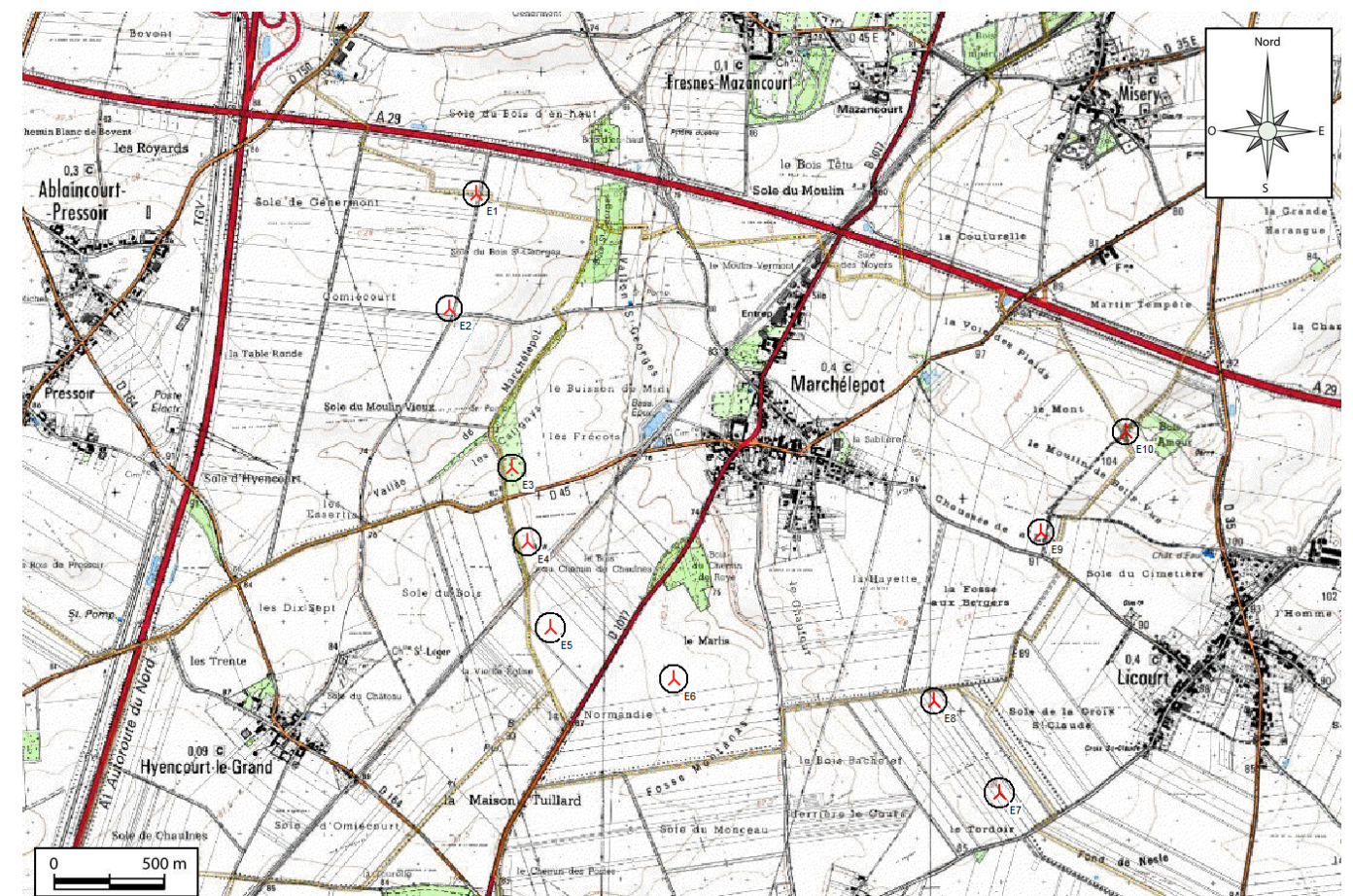
Zones d'effet des phénomènes « Chute de glace » et « Chute d'éléments de l'éolienne »
