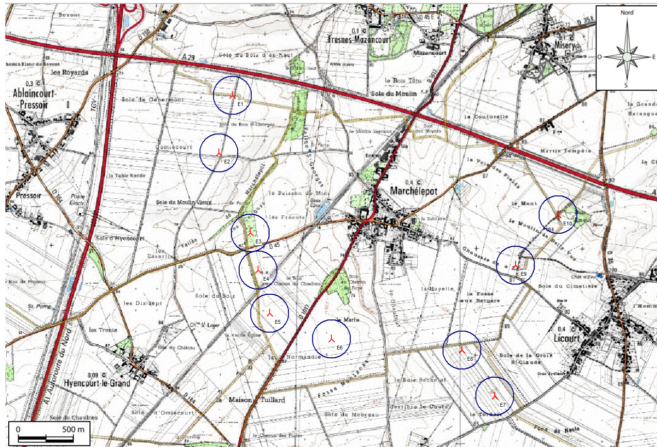
Zone d'effet du phénomène « Effondrement de l'éolienne »
