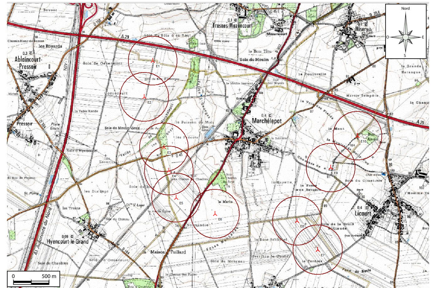
Zone d'effet du phénomène « Projection de glace »
