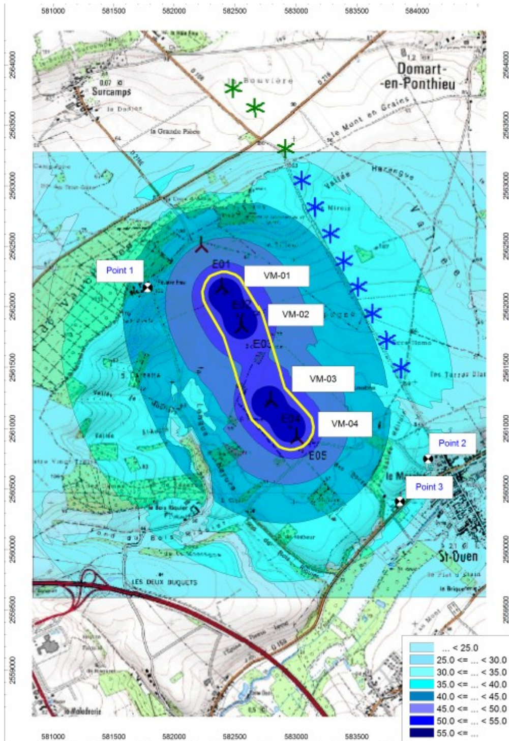
Illustration 4: Cartographie des niveaux sonores en limite de périmètre
