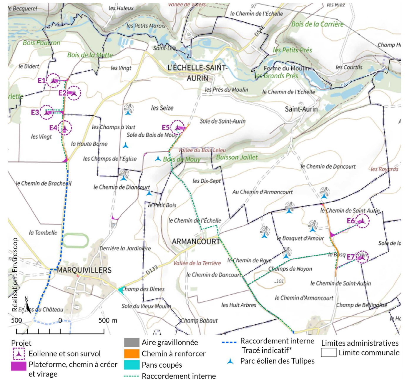
Carte 14 : Plan simplifié du parc éolien des Althéas
