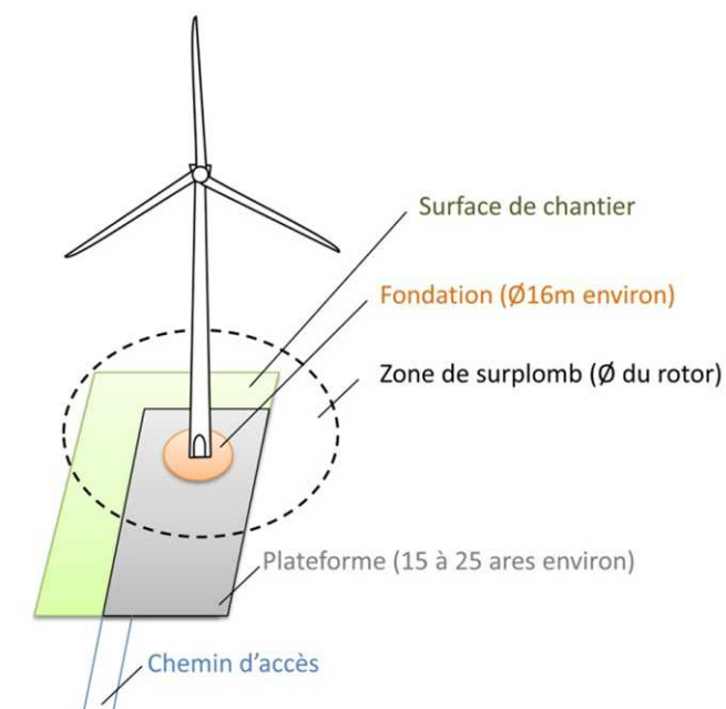
Figure 5 : schémas de principe des emprises au sol d'une éolienne
