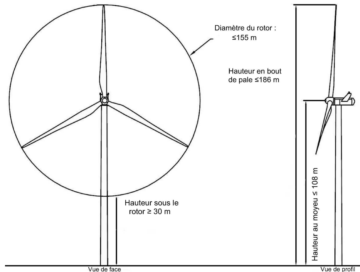
Figure 2 : Vue d'ensemble du gabarit pour les éoliennes de E1 à E6
