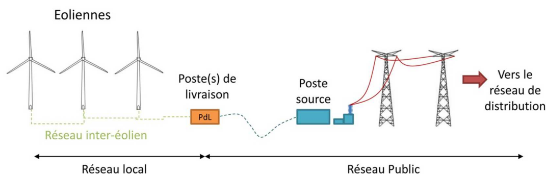
Figure 6 : Principe du raccordement électrique des installations
