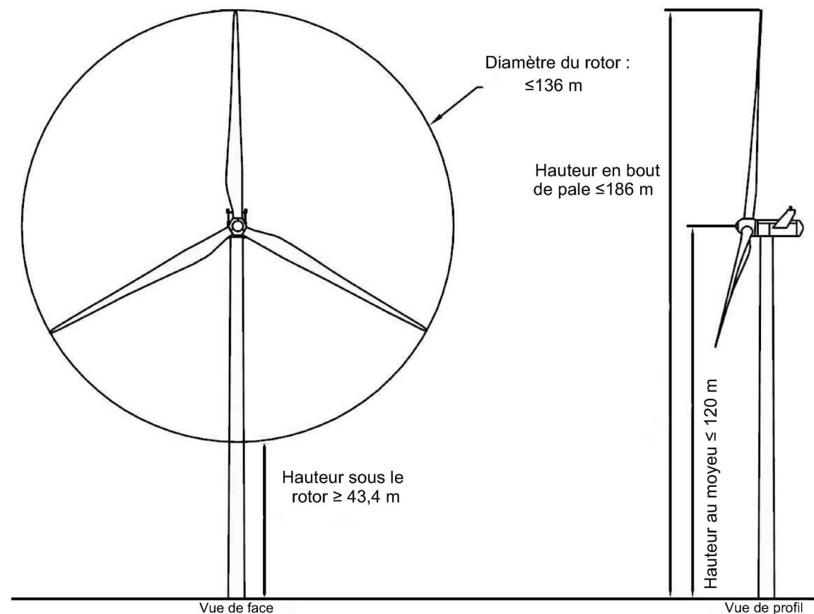
Figure 3 : Vue d'ensemble du gabarit pour l'éolienne E7
