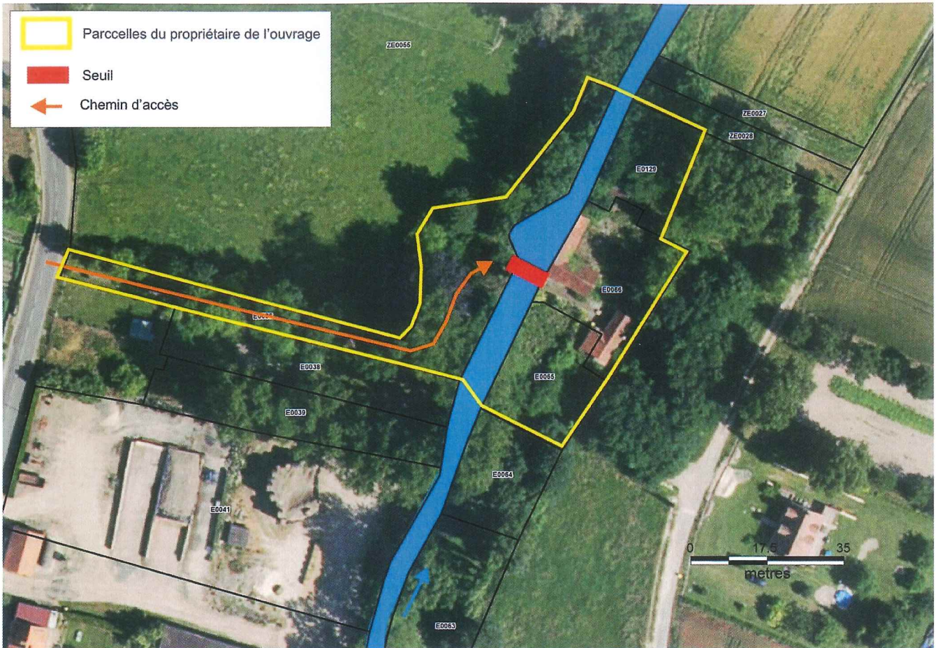
Localisation de l'ouvrage Roe 23304 (BdOrtho, Ameva).
