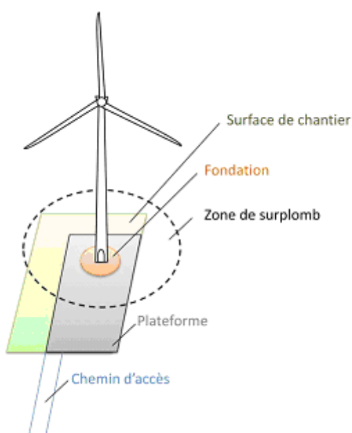
Figure 10 - Illustration des emprises au sol d'une éolienne
