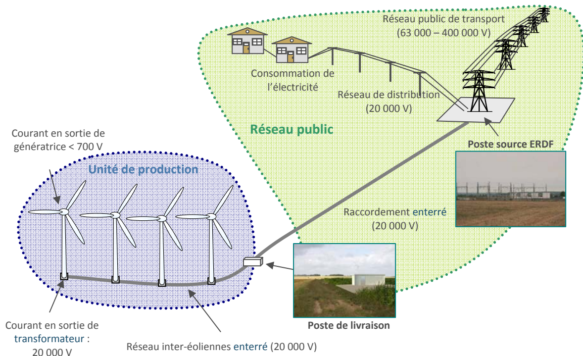
Figure 8 - Fonctionnement d'un parc éolien
