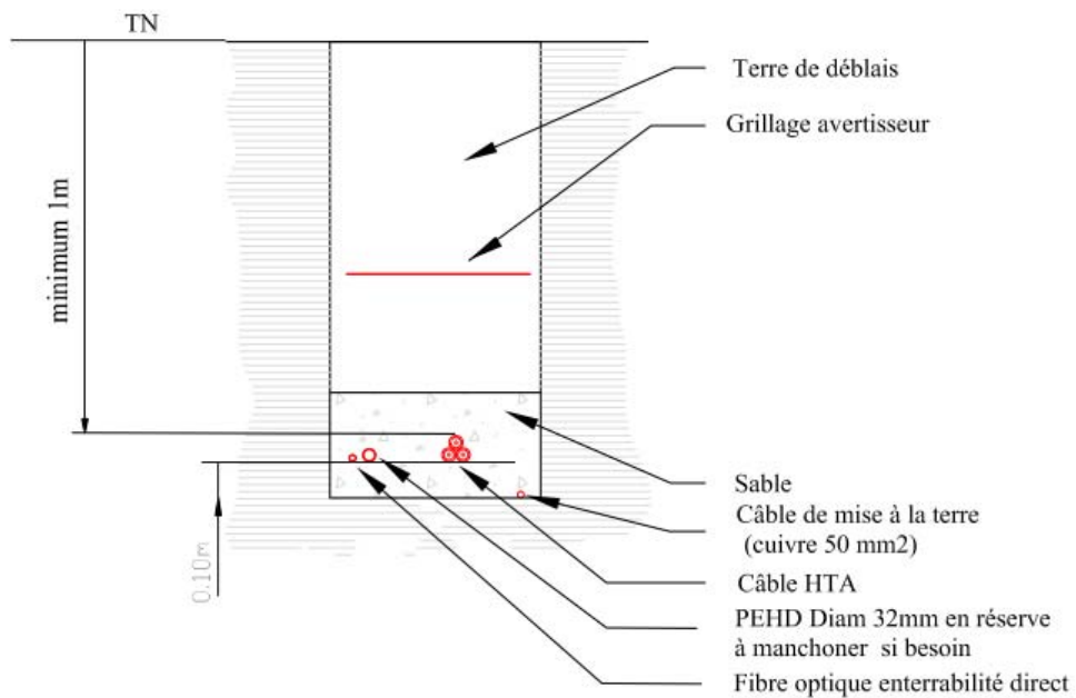
Figure 13 - Vues en coupe des tranchées
