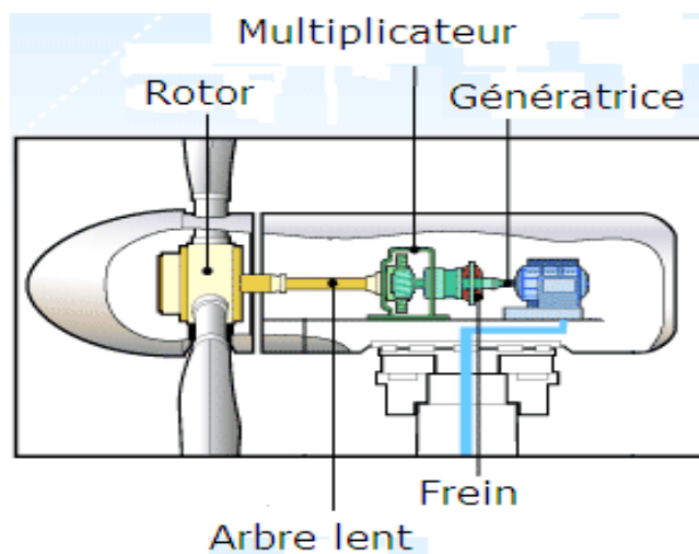
Figure 11 : Schéma simplifié de la chaîne cinématique
