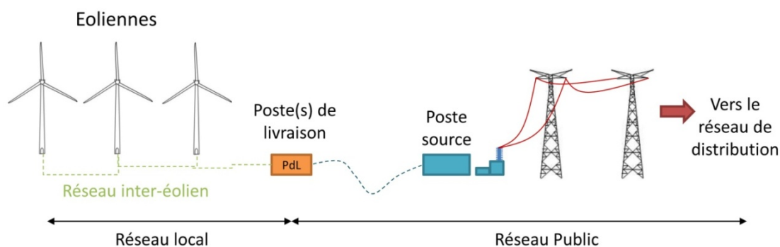
Figure 12 - Schéma de principe du raccordement électrique d'un parc éolien
