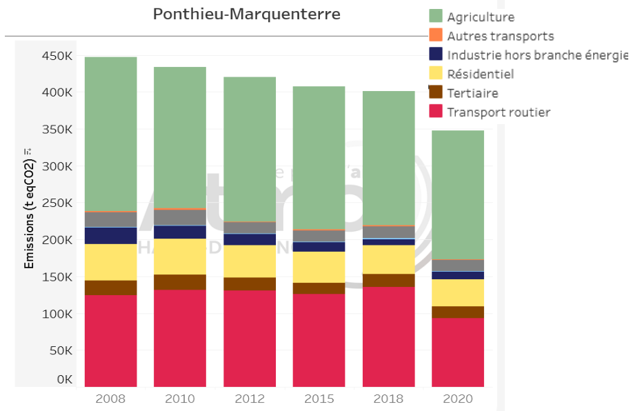
Évolution des émissions de GES par secteur PCAET - CC Ponthieu-Marquenterre
