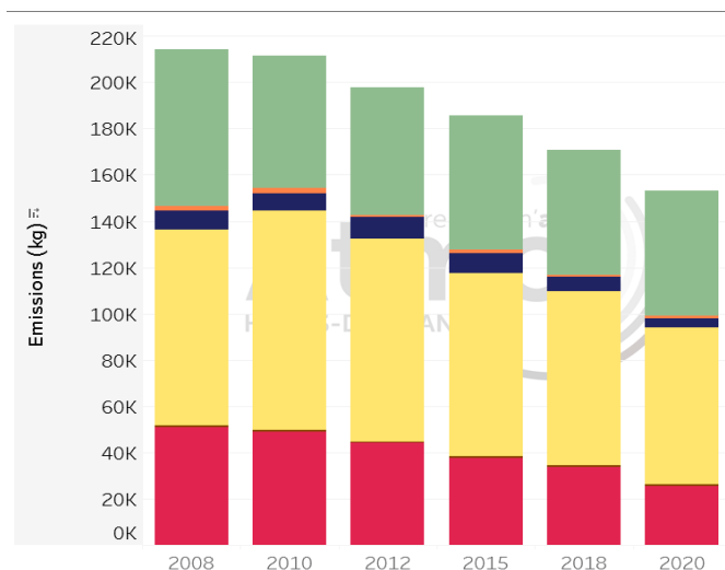
Évolution des émissions de Particules PM2.5 par secteur d'activités - CC Ponthieu-Marquenterre
